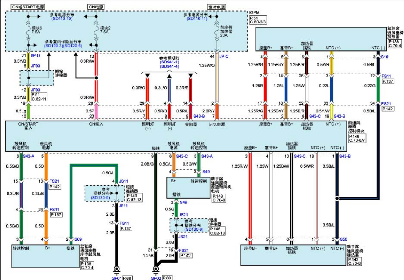
通风座椅控制系统(1)
